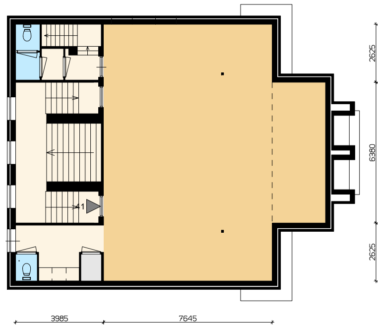
Verdieping 02
