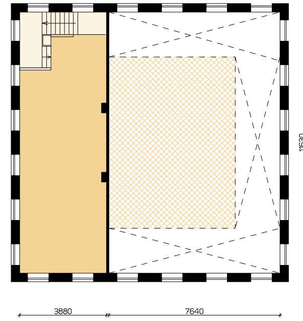
Verdieping 03
